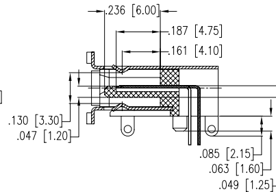
SECT A-A
