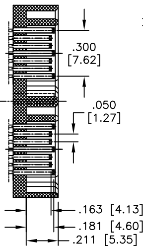
SECT A-A
