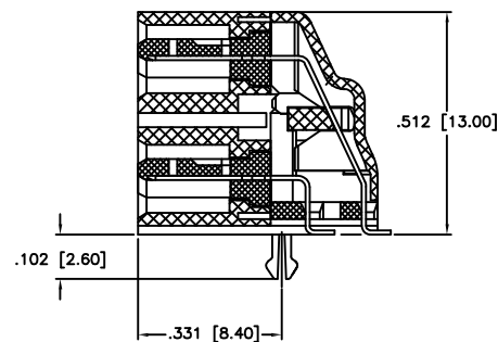
SECT A-A
