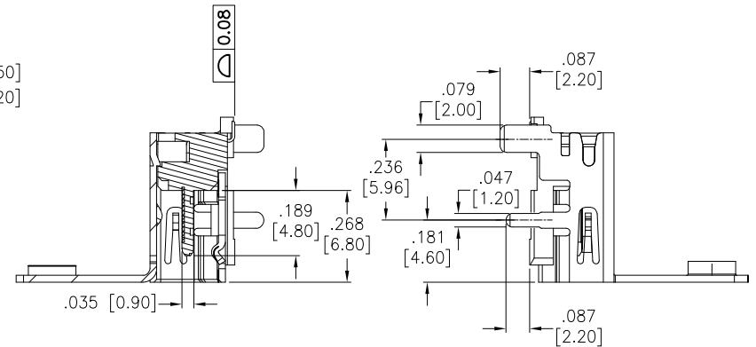
SECTION A-A SCALE 1:1
