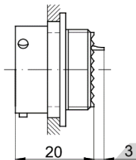
MS27497 Receptacle
