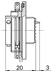
MS27513 Receptacle
