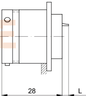
MS27505 Receptacle
