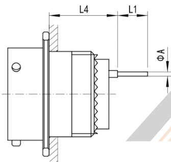
MS27472 Receptacle
