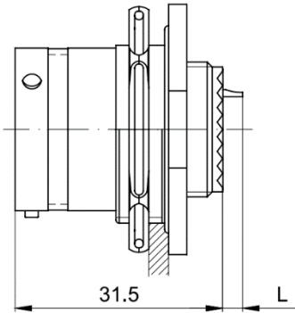
MS27468 Receptacle
