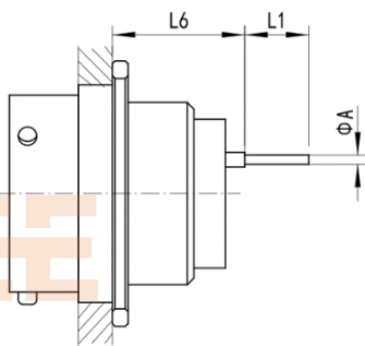
MS27508 Receptacle
