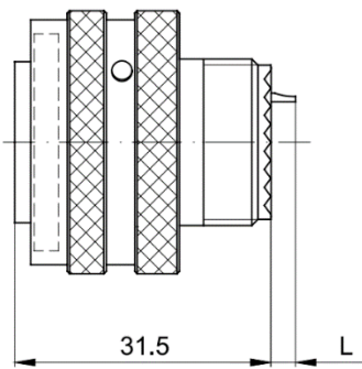
MS27656 Receptacle
