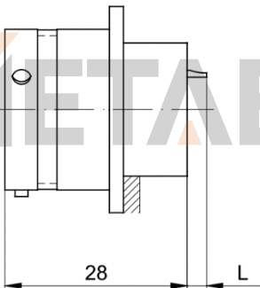
MS27496 Receptacle
