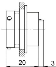
MS27508 Receptacle
