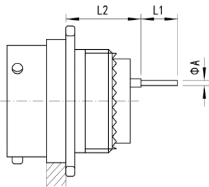
MS27513 Receptacle
