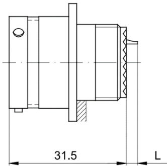
MS27505 Receptacle
