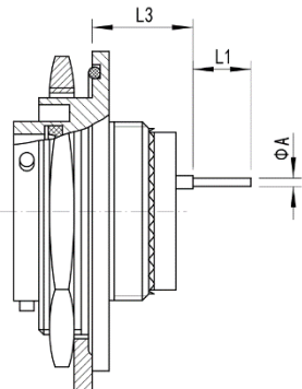
MS27508 Receptacle
