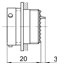
MS27508 Receptacle
