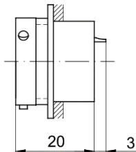
MS27513 Receptacle
