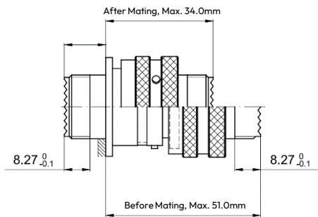
MS27496 Receptacle / MS27467 Plug
