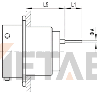
MS27513 Receptacle
